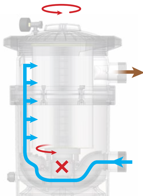
Il flusso d'acqua durante il controlavaggio
