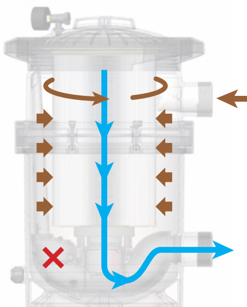
Il flusso d'acqua durante la filtrazione
